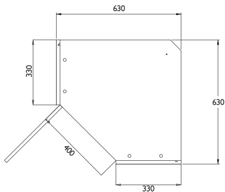
1450 630W Corner Wall 400W Door
