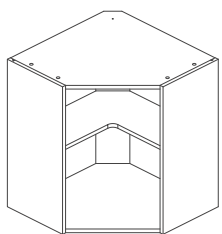
1450 630W Corner Wall 400W Door
