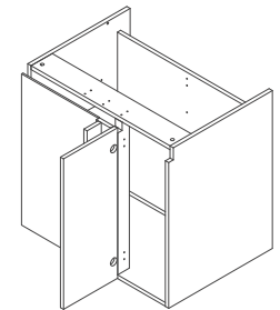
RH Unit, LH Blank
